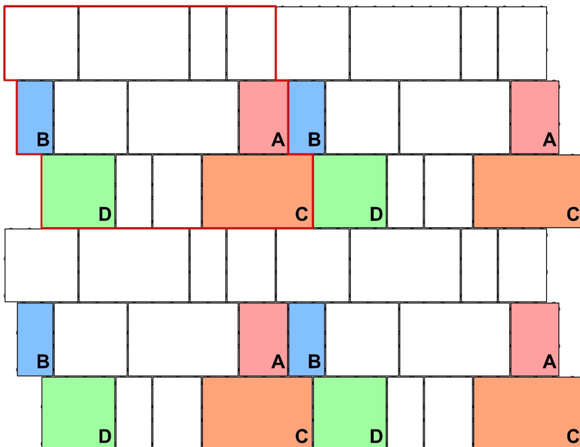
Obr. č. 4 – Rozložení čtyř vrstev a narušení spár výměnou kamenů
