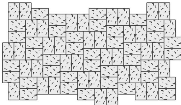
Obr. č.3 – Návrh pokládky z prvků Obdélník 18 / 12 / 4
