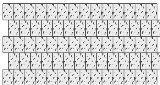
Obr. č.4 – Návrh pokládky z prvků Obdélník 18 / 12 / 4
