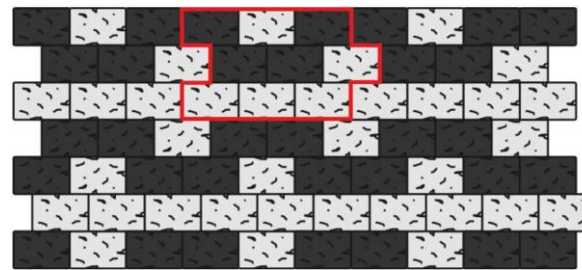
Obr. č.10 – Návrh pokládky z prvků Obdélník 21 / 14 / 7 History
