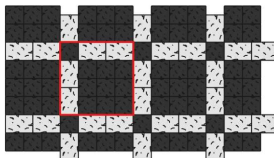
Obr. č.18 – Návrh pokládky z prvků Obdélník 21 / 14 / 7 History a Čtverec 14 / 14 / 7 History
