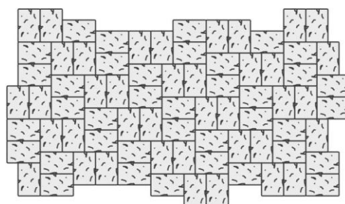
Obr. č.12 – Návrh pokládky z prvků Obdélník 21 / 14 / 7 History
