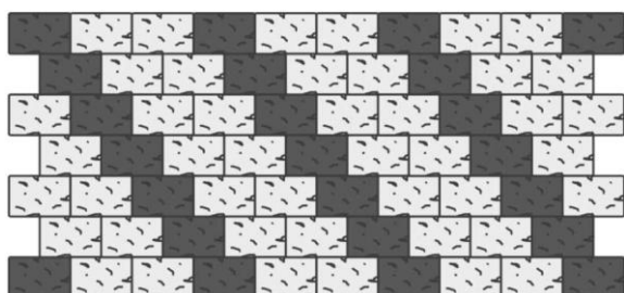
Obr. č.9 – Návrh pokládky z prvků Obdélník 21 / 14 / 7 History
