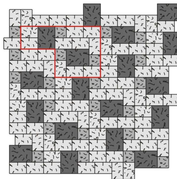
Obr. č.20 – Návrh pokládky z prvků Obdélník 28 / 21 / 7, Obdélník History, 21 / 14 / 7 History a Čtverec 14 / 14 / 7 History
