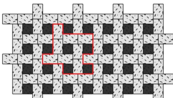
Obr. č.17 – Návrh pokládky z prvků Obdélník 21 / 14 / 7 History a Čtverec 14 / 14 / 7 History
