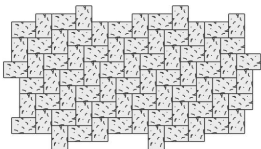
Obr. č.11 – Návrh pokládky z prvků Obdélník 21 / 14 / 7 History
