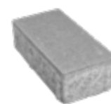
PARKETA 6 ROVNÁ HRANA Rozměry: 20 × 10 × 6 cm
