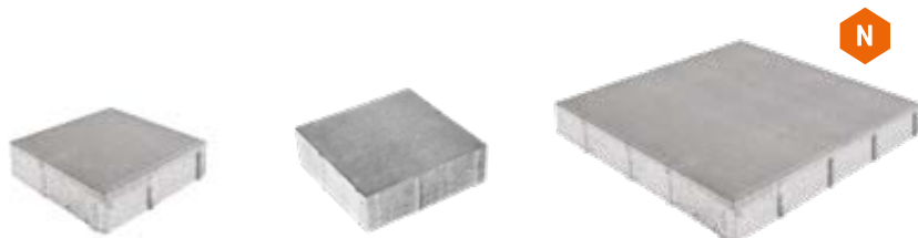
KOSTKA 6 Rozměry: 20 × 20 × 6 cm KOSTKA 8 Rozměry: 20 × 20 × 8 cm
